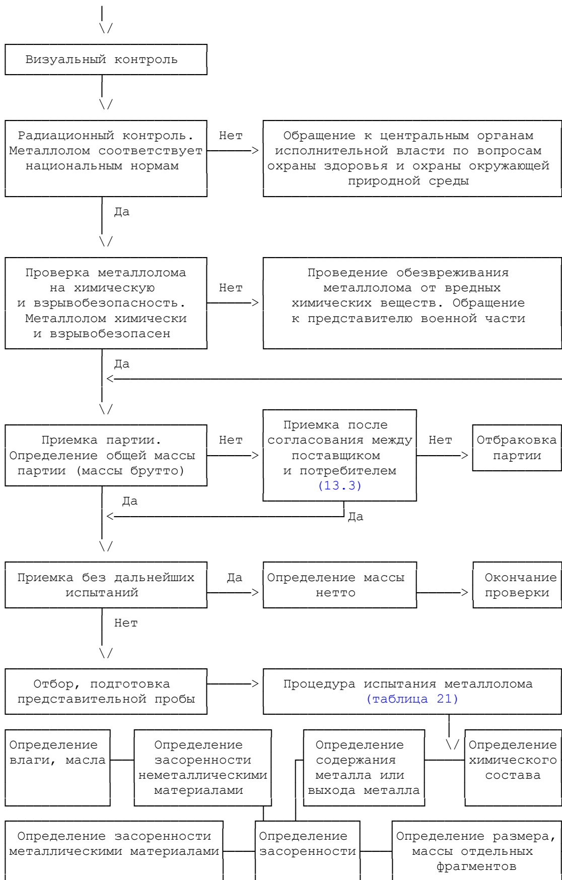
Рисунок 1. Схема проверки поступающего металлолома
